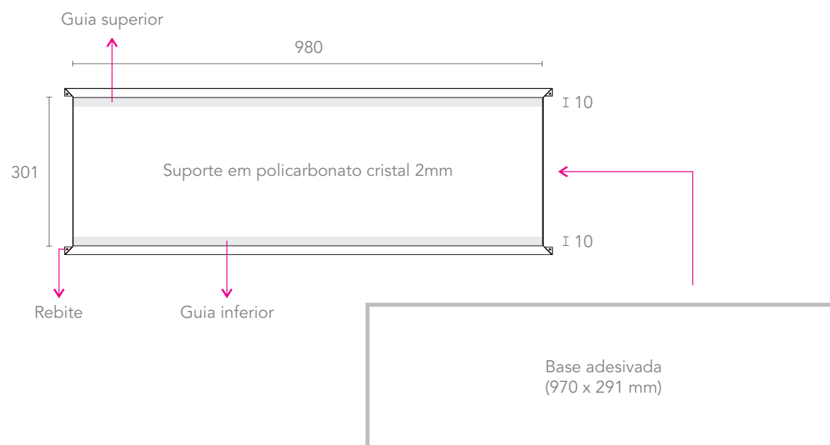
Vista lateral em detalhe (corte transversal AA)
