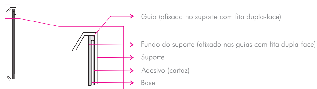
Vista lateral em detalhe (corte transversal AA)
