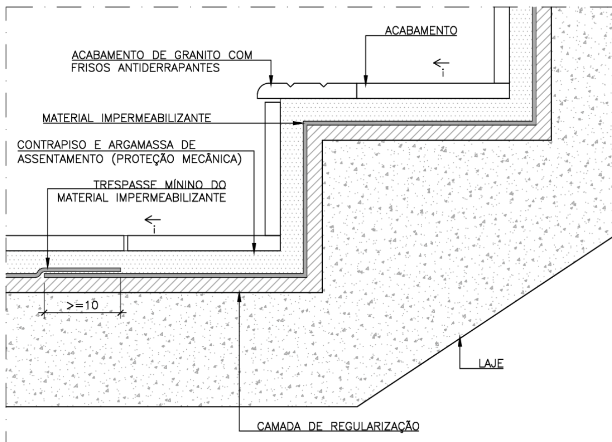
DETALHE – IMPERMEABILIZAÇÃO DE DEGRAUS DE ESCADA SEM ESCALA
