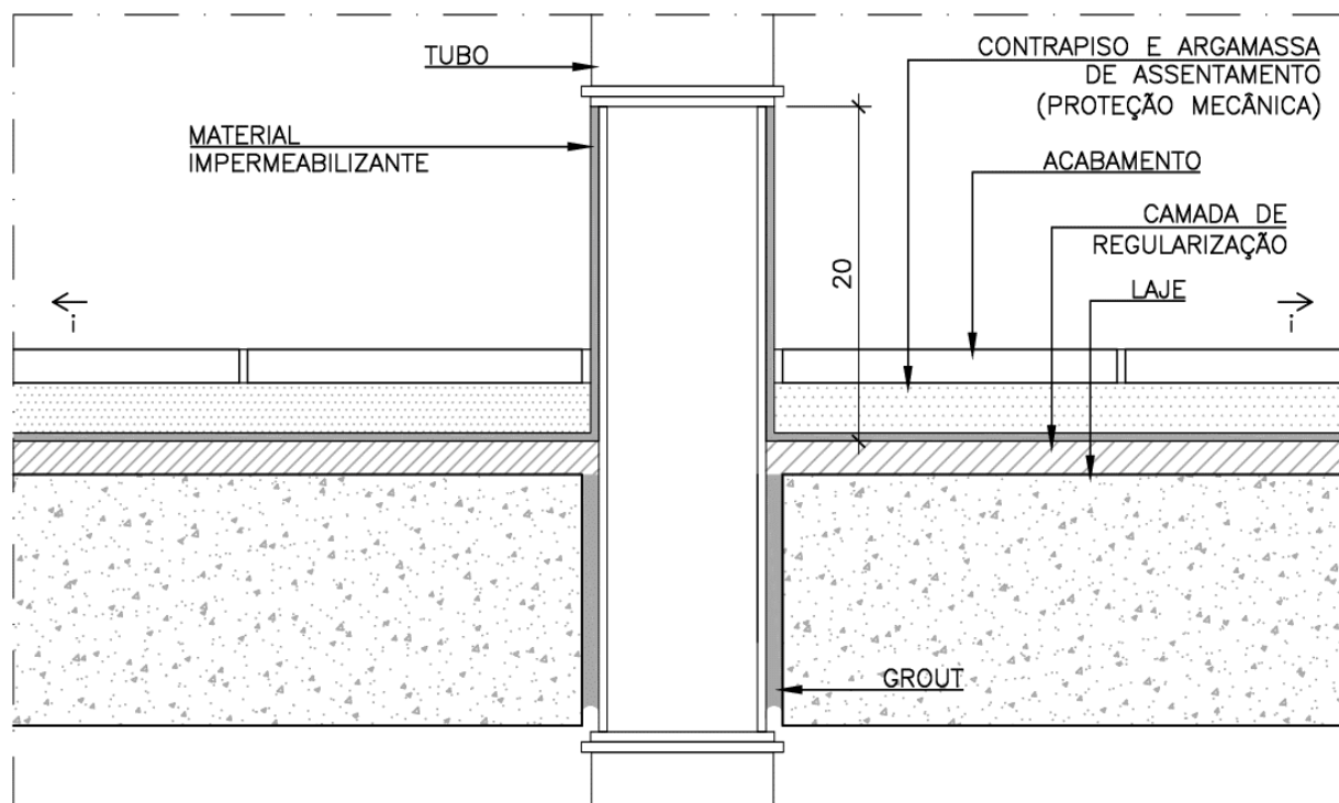
DETALHE – IMPERMEABILIZAÇÃO DE TUBO PASSANTE SEM ESCALA
