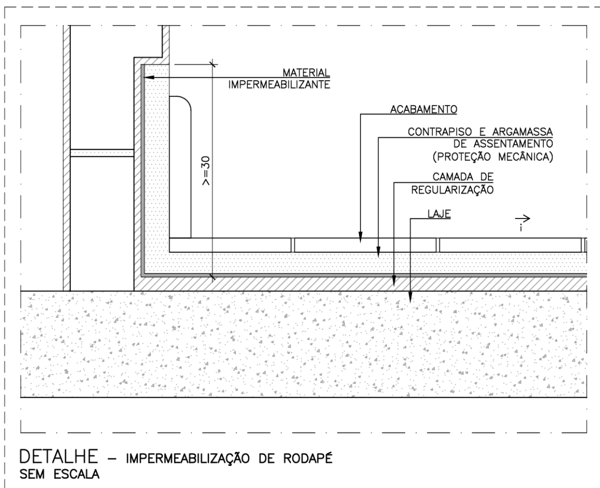
Figura 1 - Detalhe da impermeabilização de rodapés
