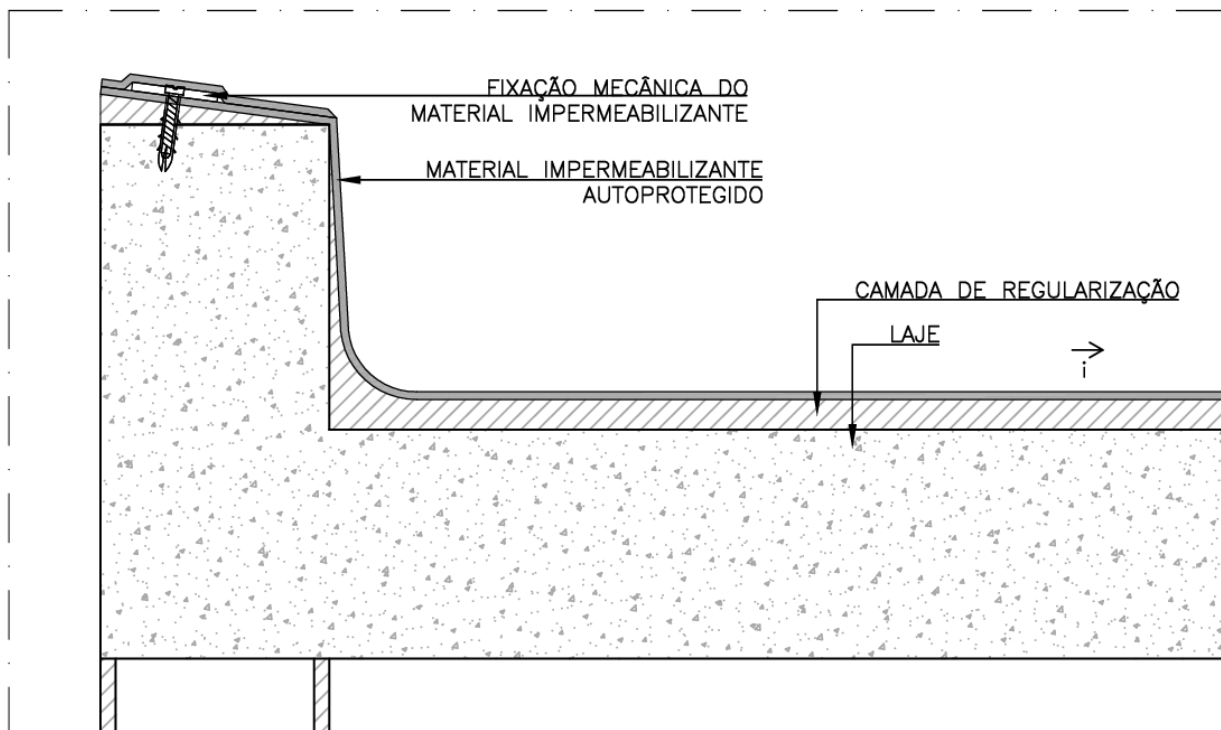
DETALHE – ARREIMATE DE IMPERMEABILIZAÇÃO DE BORDA DE LAJE SEM ESCALA
