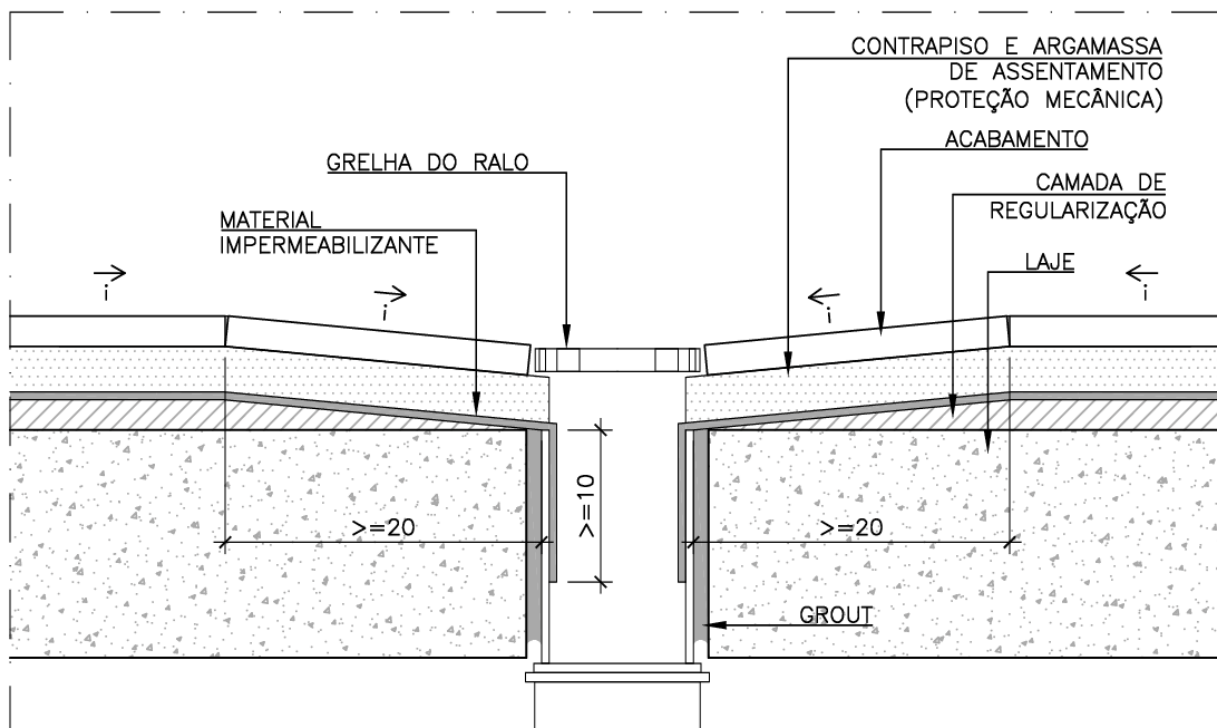
DETALHE – IMPERMEABILIZAÇÃO DE RALO SEM ESCALA
