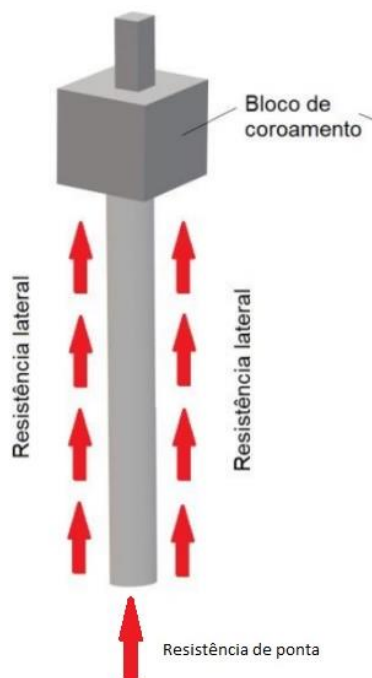
Figura 1 - Desenho esquemático com esquema de estaca. Fonte: Elaboração própria.
