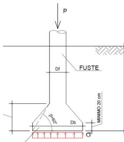
Figura 2 - Desenho esquemático com esquema de tubulão. Fonte: Elaboração própria.
