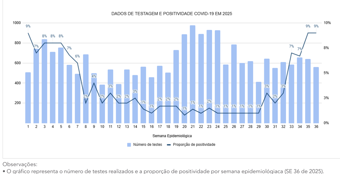
GRÁFICO 7 Testes realizados para Covid-19, segundo semana epidemiológica da data de coleta. Belo Horizonte, 2025.
