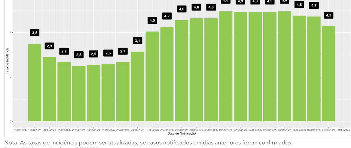
GRÁFICO 1 Incidência de COVID-19, acumulada nos últimos 14 dias, por 100.000 habitantes.
