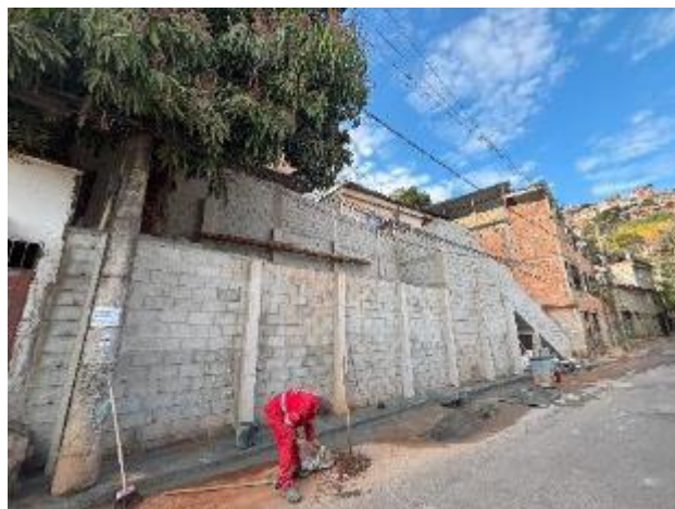
Obra de muro de contenção, drenagem e escada de acesso Rua Nossa Senhora de Fátima, 1400 Vila Nossa Senhora de Fátima – Centro Sul
