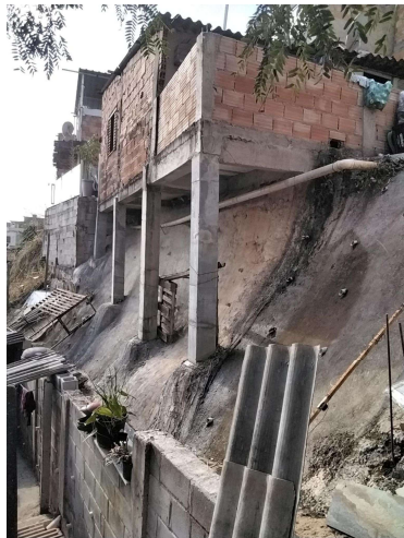
Obra de Contenção, tratamento de encosta R. Maria Camargo Diniz, 15 - Ventosa - antes e depois da obra
