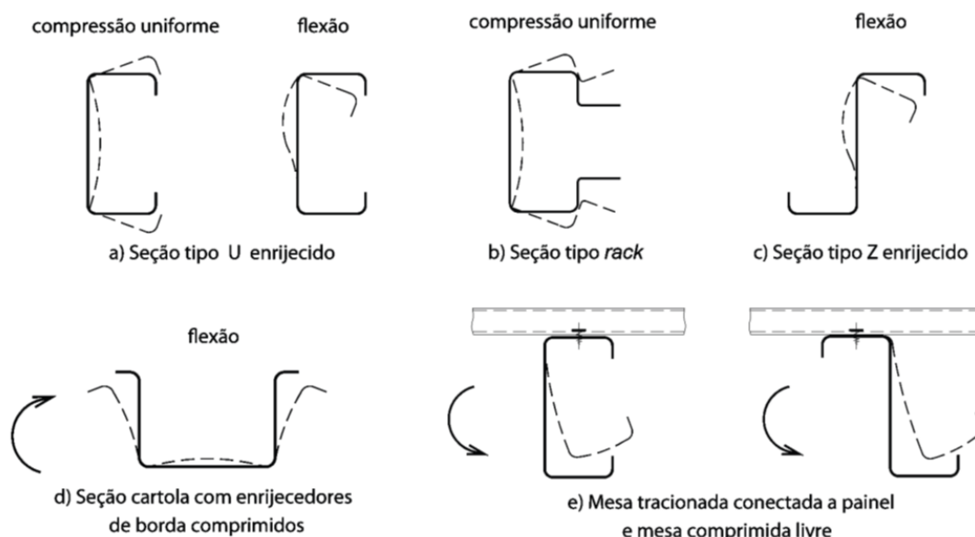
Figura 25.2 - Flambagens distorcionais da seção transversal. Fonte: ABNT (2010).
