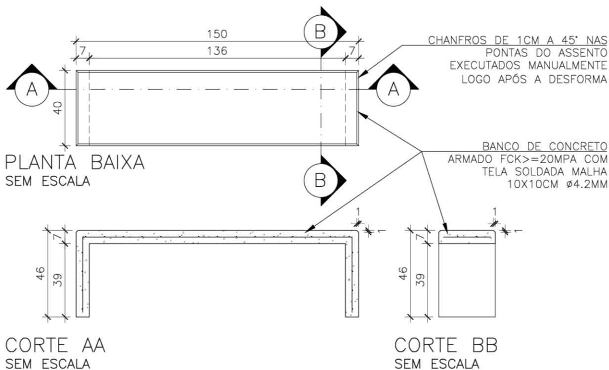
Figura 9 - Banco 150 cm de concreto moldado in loco. Elaboração própria. Nota: Desenho elaborado em 21/07/2025.
