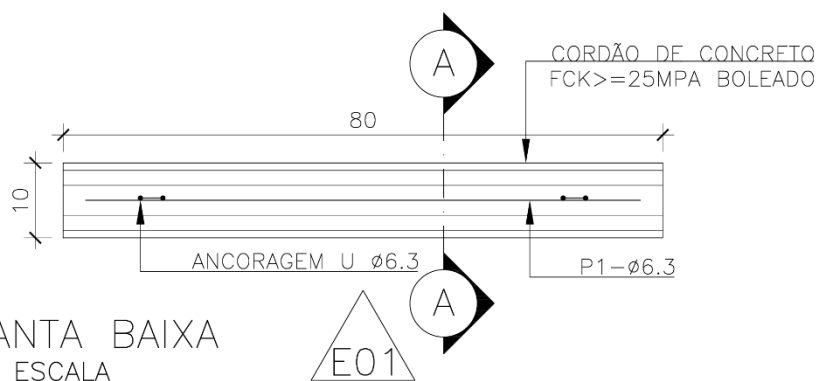
Figura 21 - Cordão de concreto boleado altura 5 cm. Elaboração própria. Nota: Desenho elaborado em 21/07/2025.
