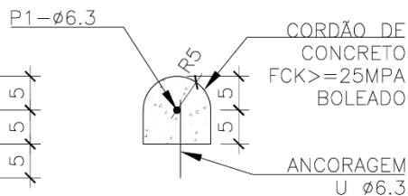
CORTE AA SEM ESCALA
