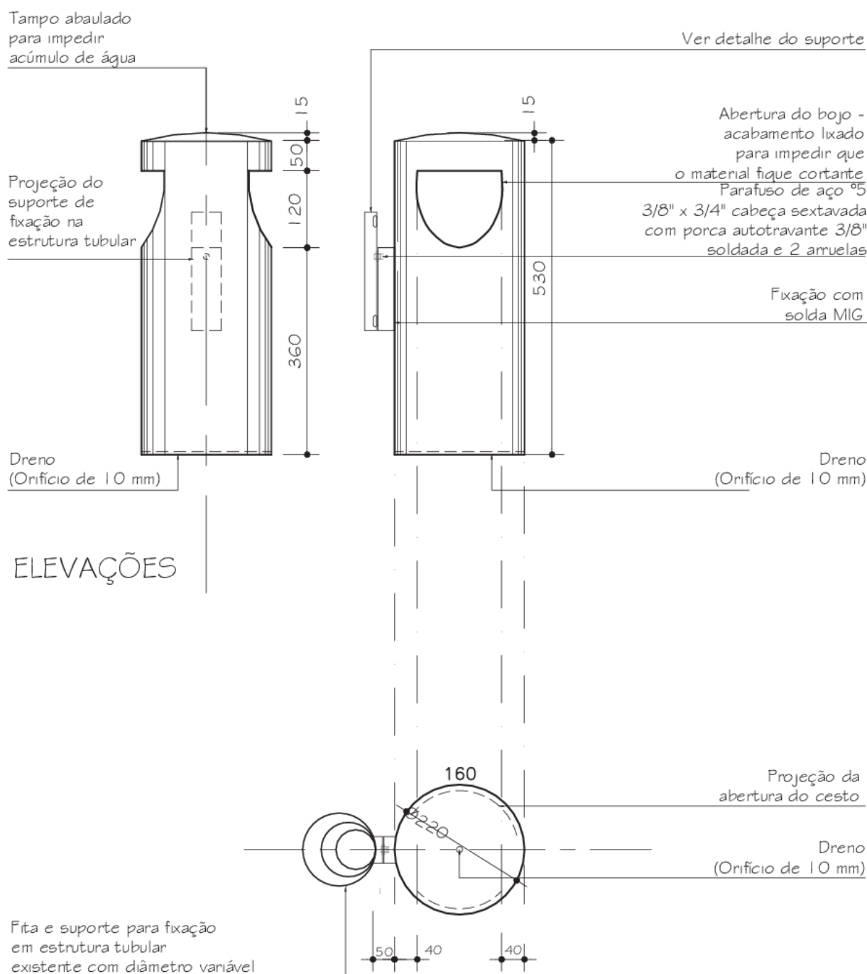
Figura 29 - Cesto coletor de resíduo leve MC22. Fonte: SLU (2019).
