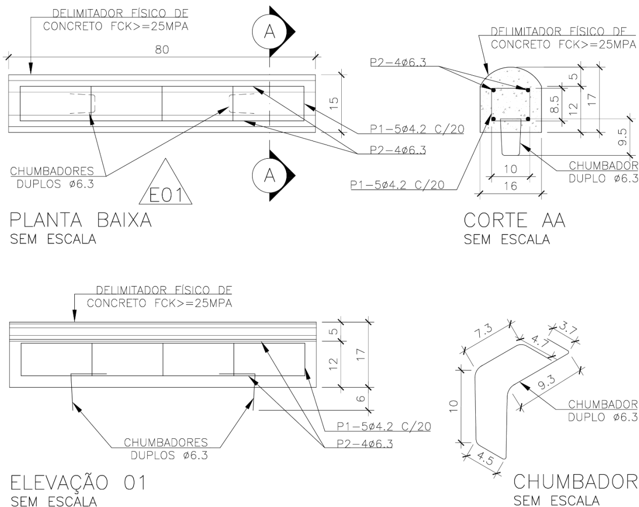
Figura 23 - Delimitador físico de concreto. Elaboração própria. Nota: Desenho elaborado em 21/07/2025.
