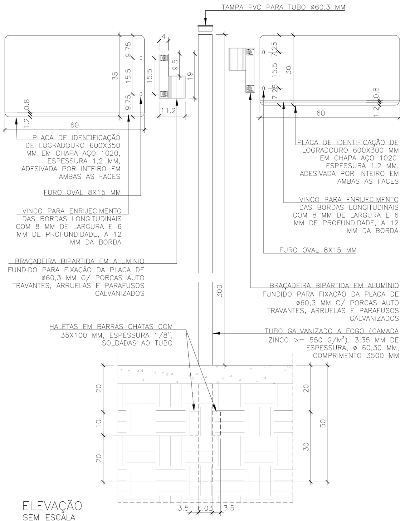
Figura 6 - Elevação placa de identificação de logradouro com vinco e adesivada por inteiro tipo altura 30 cm e tipo altura 35 cm. Elaboração própria. Nota: Desenho elaborado em 03/11/2025.
