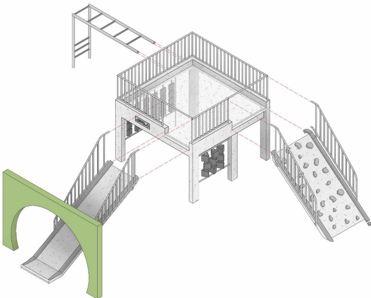
Figura 38 - Playground padronizado - Módulo escorregador (independente). Fonte: Elaboração própria. Nota: Desenho elaborado em 21/07/2025.
