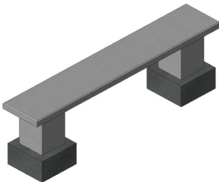
Figura 8 - Imagem 3D do Banco de placa de concreto apoiado. Elaboração própria. Nota: Desenho elaborado em 21/07/2025.
