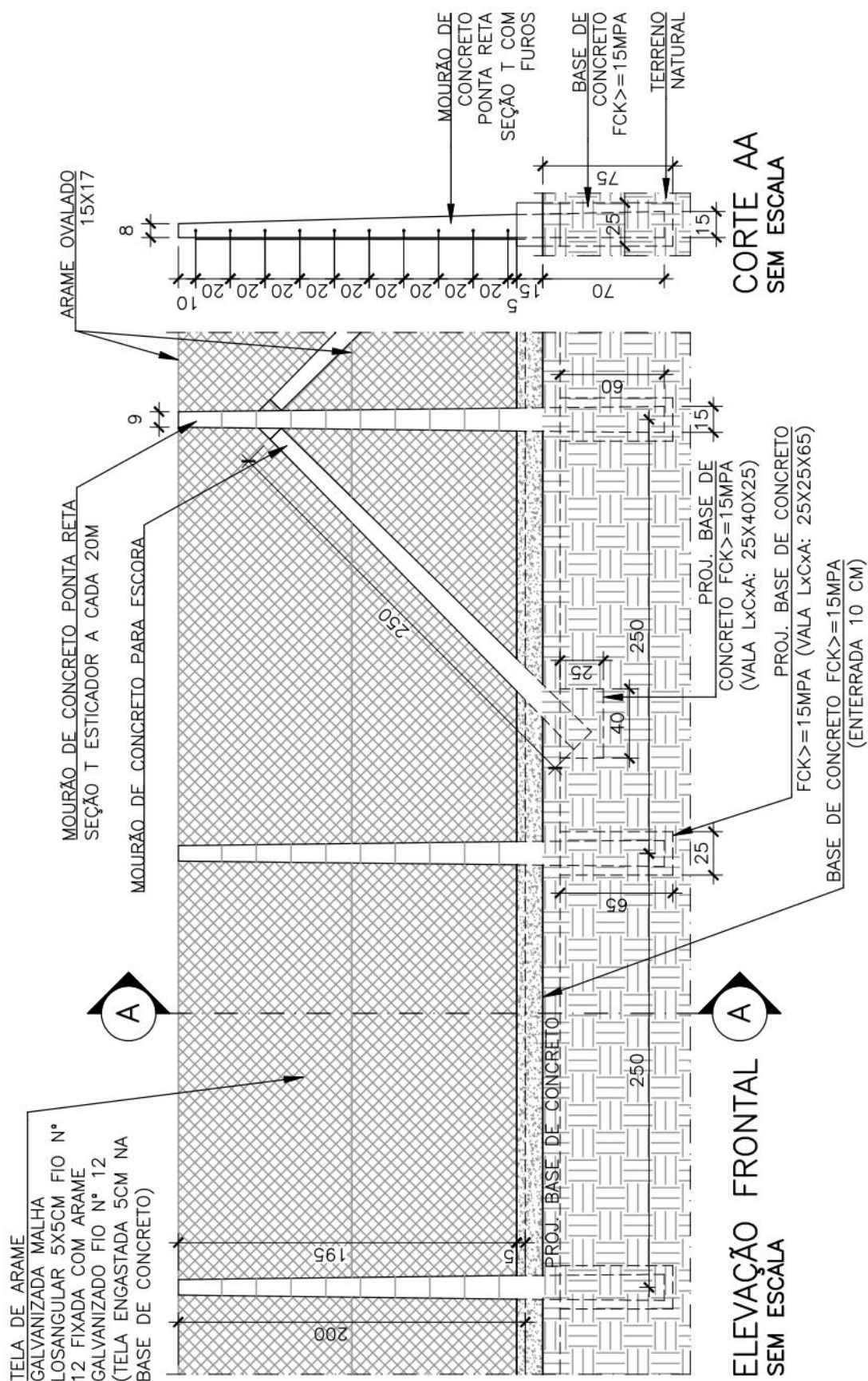
Figura 24 - Cerca com mourões de concreto ponta reta e tela galvanizada. Elaboração própria. Nota: Desenho elaborado em 28/09/2022.
