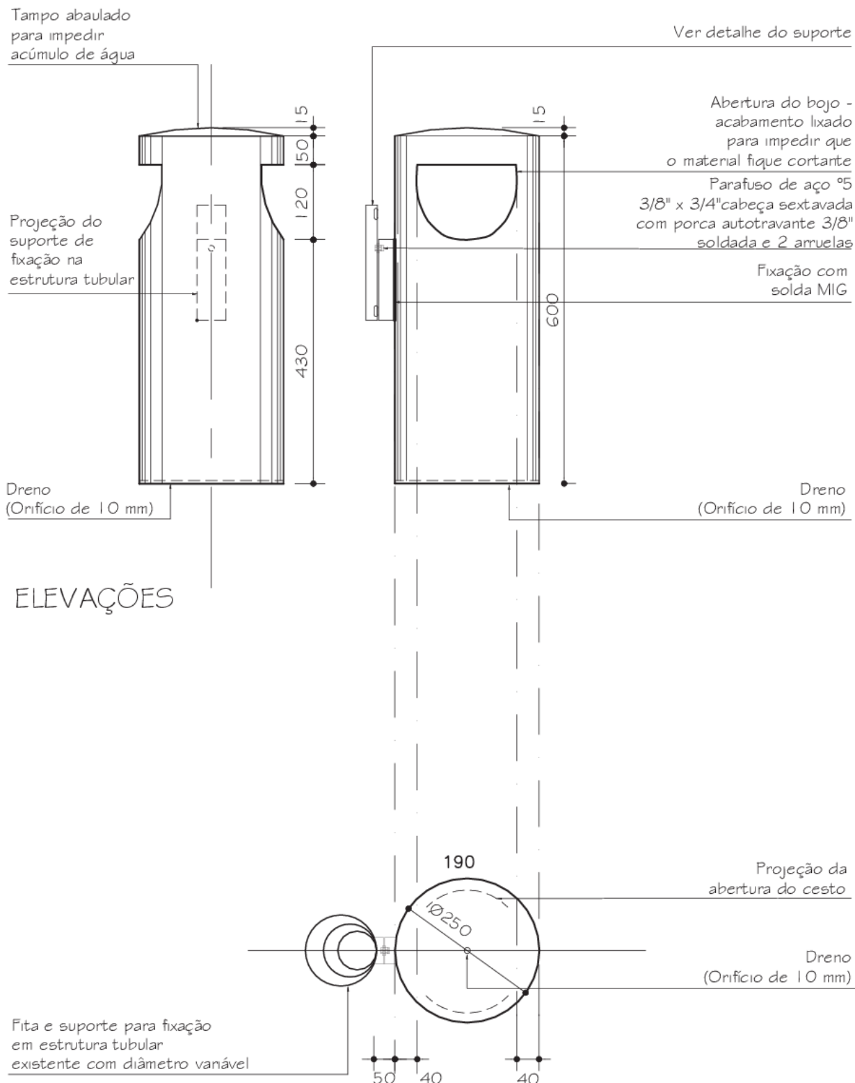
Figura 30 - Cesto coletor de resíduo leve MC25. Fonte: SLU (2019).
