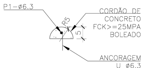
CORTE AA SEM ESCALA
