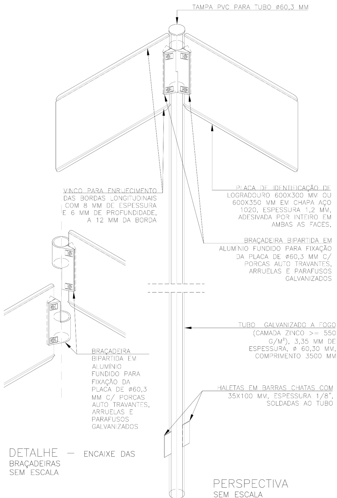
Figura 5 - Perspectiva da placa de identificação de logradouro com vinco e adesivada por inteiro. Elaboração própria. Nota: Desenho elaborado em 03/11/2025.
