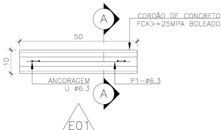
PLANTA BAIXA SEM ESCALA
