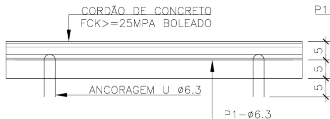
ELEVAÇÃO 01 SEM ESCALA
