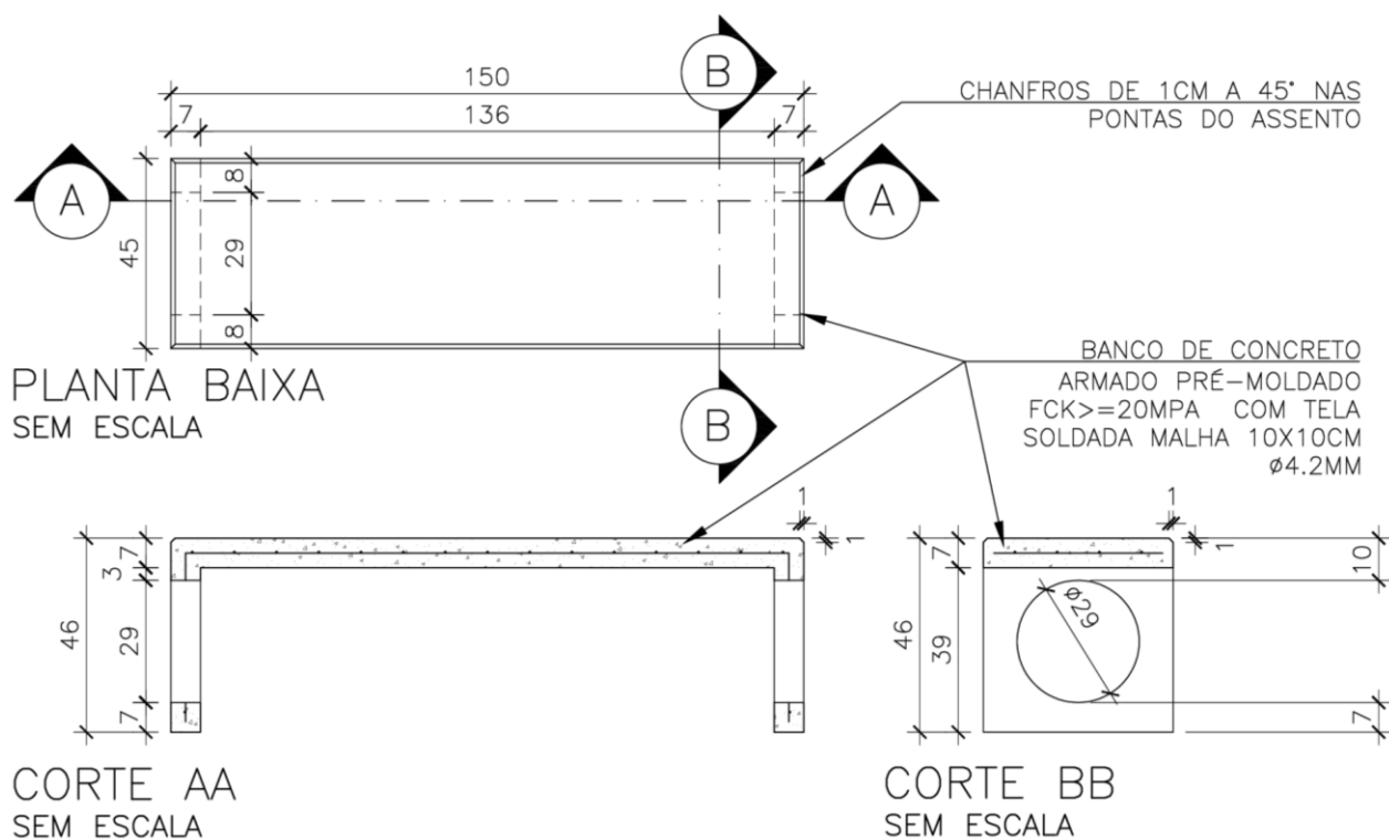
Figura 11 - Banco de concreto pré-fabricado. Elaboração própria. Nota: Desenho elaborado em 21/07/2025.
