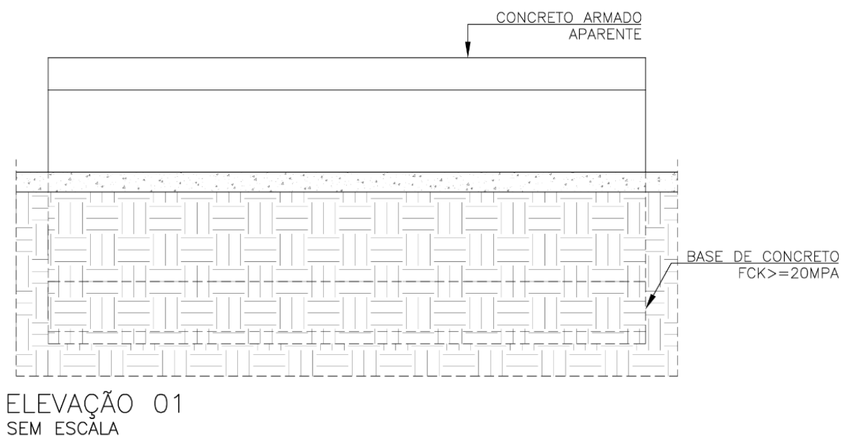
Figura 15 - Banco linear delimitador de concreto. Elaboração própria. Nota: Desenho elaborado em 21/07/2025.
