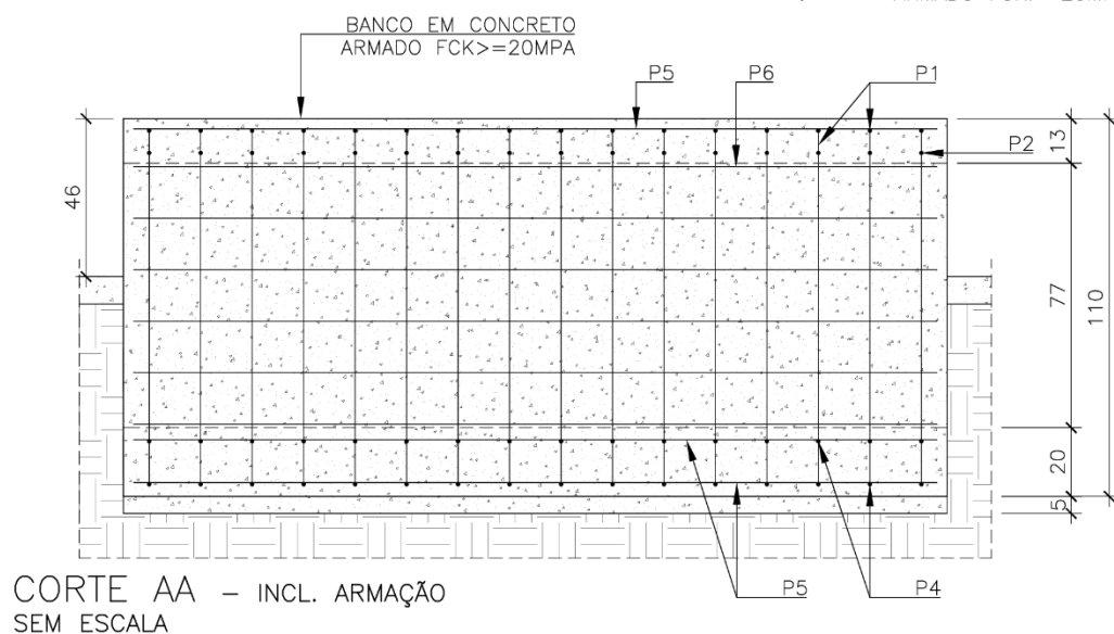
Figura 16 - Banco linear delimitador de concreto. Elaboração própria. Nota: Desenho elaborado em 21/07/2025.
