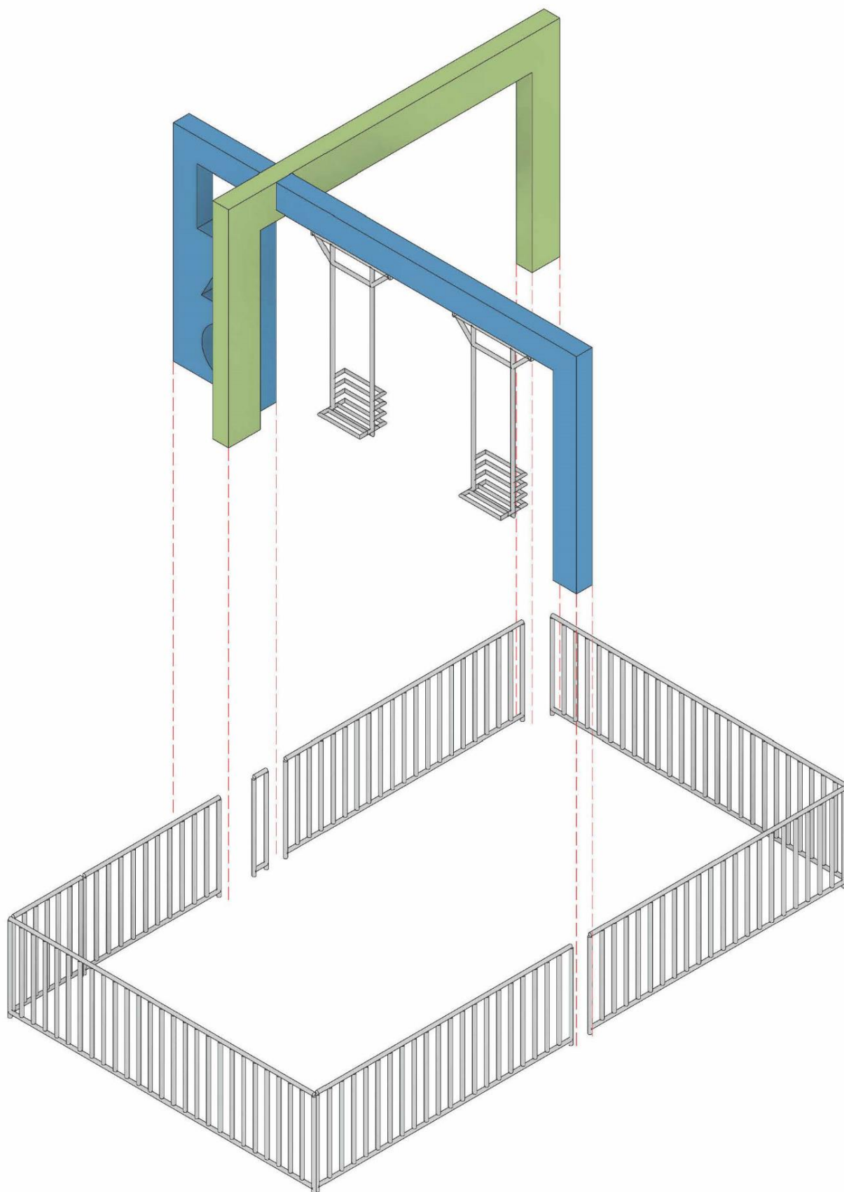
Figura 39 - Playground padronizado - Módulo balanço (dependente). Fonte: Elaboração própria. Nota: Desenho elaborado em 21/07/2025.
