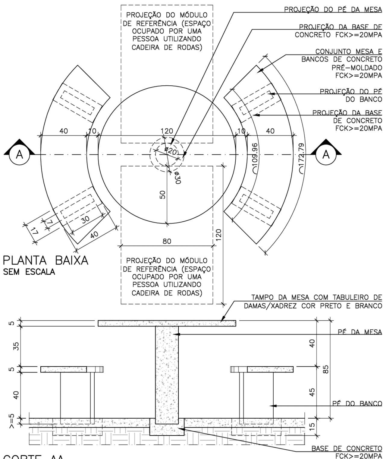
Figura 19 - Conjunto acessível de concreto pré-fabricado de mesa para jogos e 2 bancos. Elaboração própria. Nota: Desenho elaborado em 12/12/2019.
