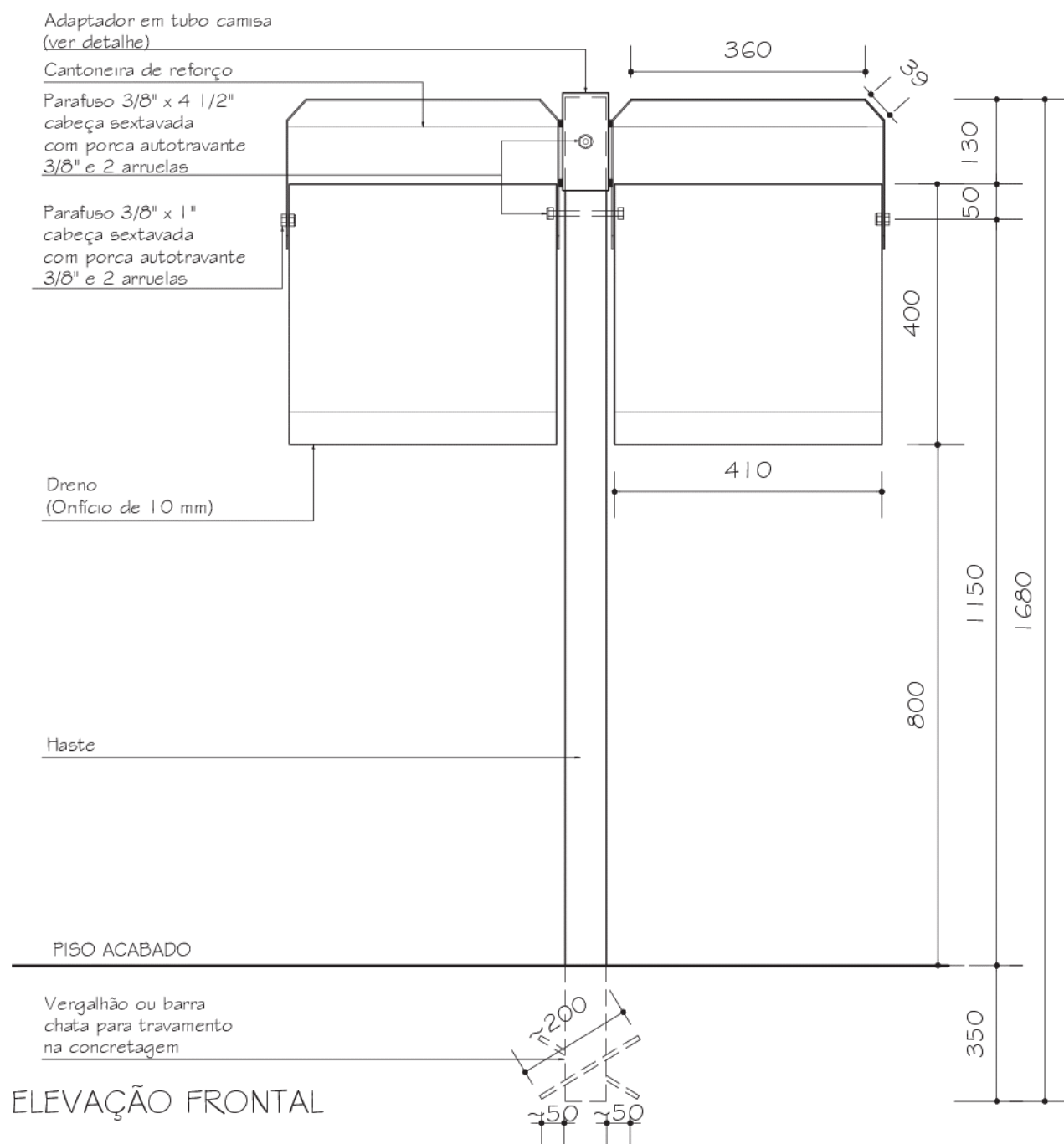
Figura 33 - Cesto coletor de resíduo leve MQD - Elevação Frontal. Fonte: SLU (2019).
