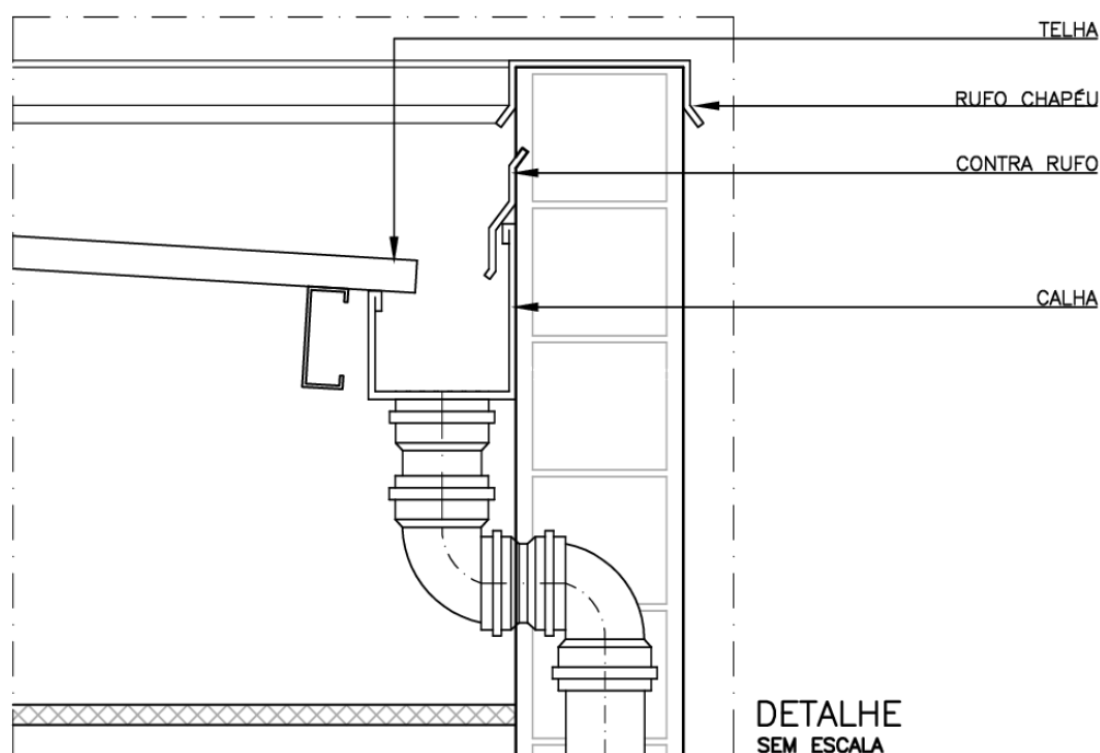
Figura 11 - Interligação da calha / Condutor vertical. Fonte: Elaboração própria. Nota: Desenho elaborado em 10/03/2023.
