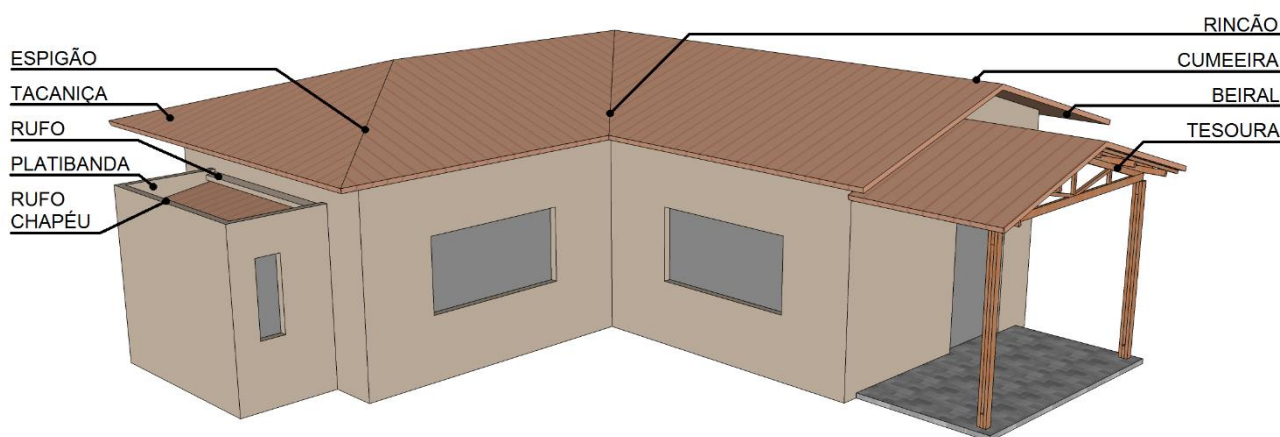
Figura 1 - Designações da cobertura. Fonte: Elaboração própria. Nota: Desenho elaborado em 30/07/2018.
