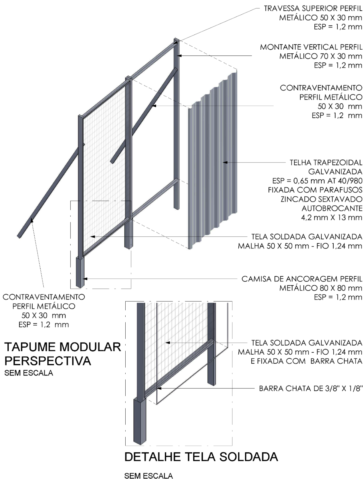
Figura 47 - Tapume modular - detalhes. Fonte: Elaboração própria. Nota: Desenho elaborado em 23/12/2025.
