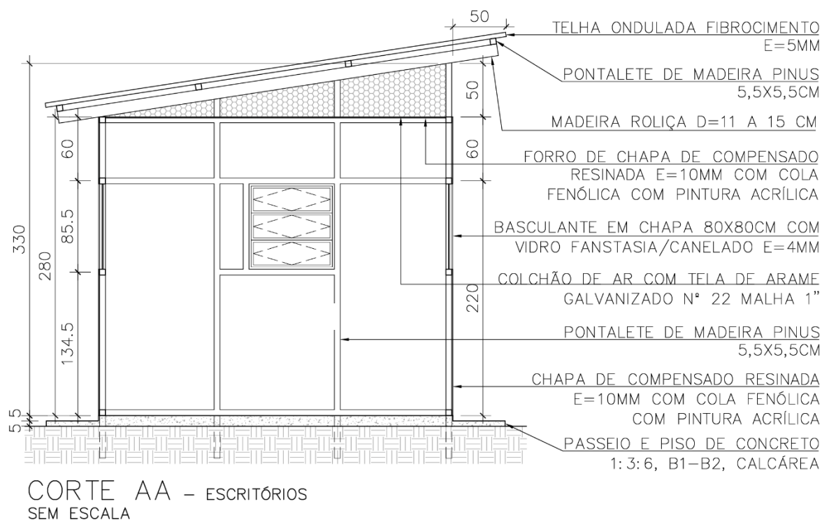
Figura 8 - Corte transversal dos escritórios de até 15 m 2 e até 22 m 2 . Fonte: Elaboração própria. Nota: Desenho elaborado em 27/09/2024.
