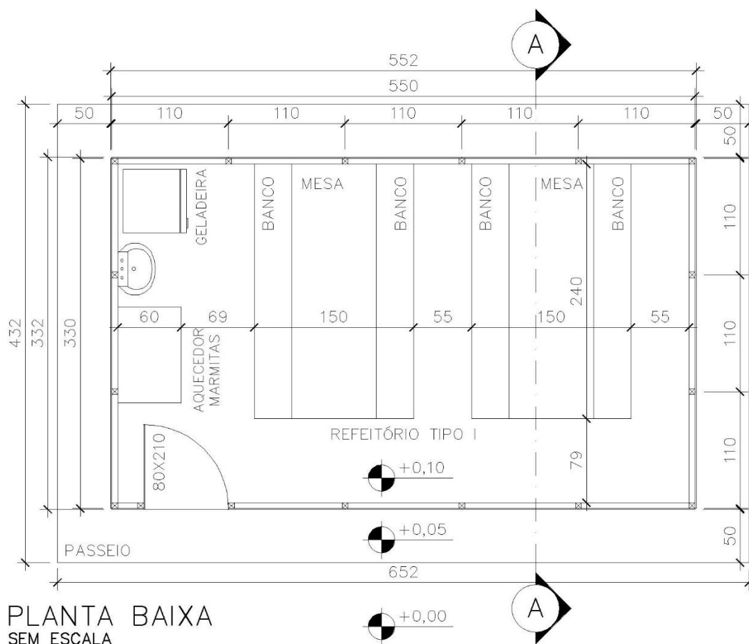
Figura 24 - Refeitório até 19 m². Fonte: Elaboração própria. Nota: Desenho elaborado em 03/07/2026.
