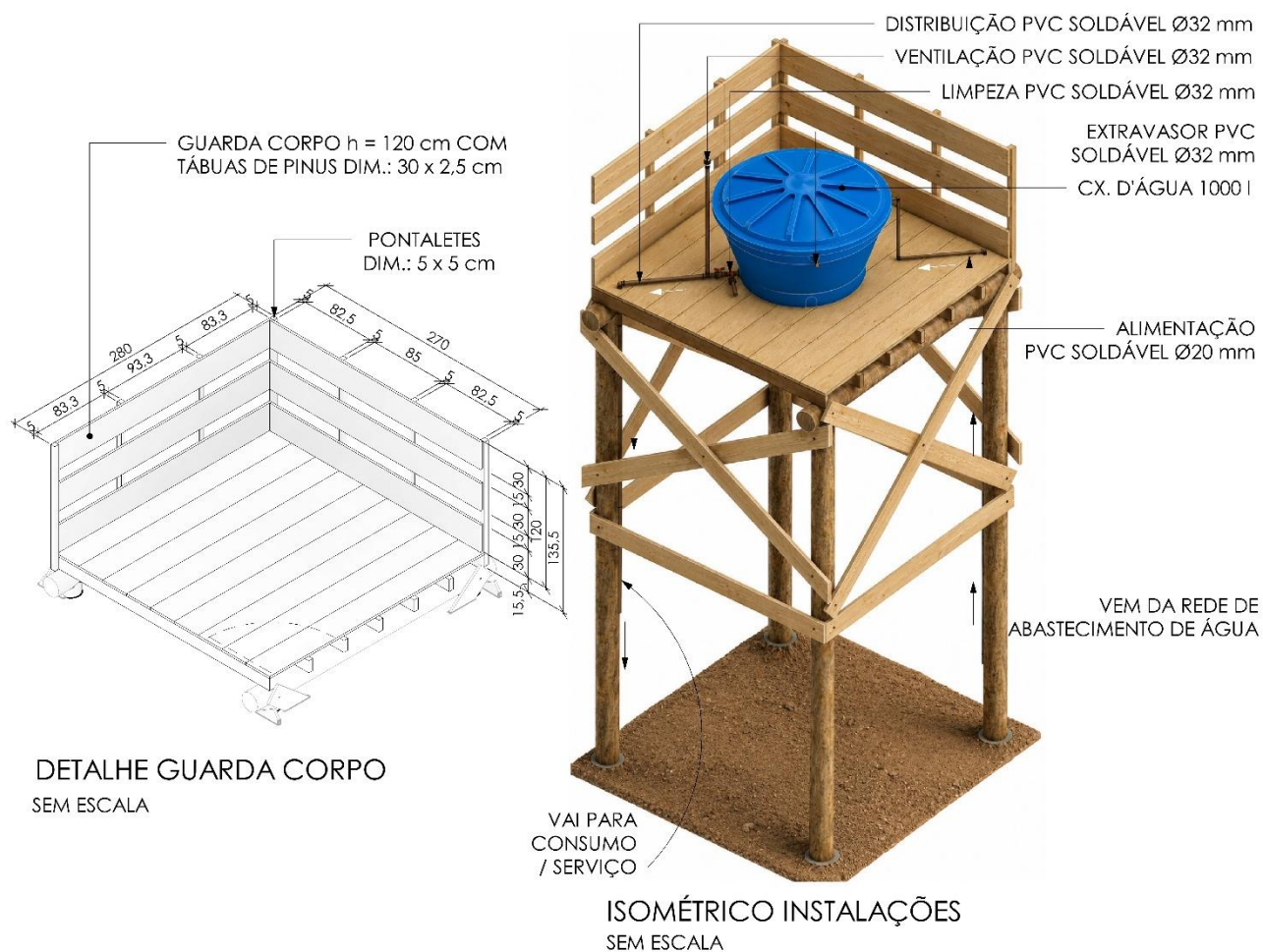
Figura 37 - Detalhe guarda corpo da torre de caixa d'água provisória. Fonte: Elaboração própria. Nota: Desenho elaborado em 03/07/2026.
