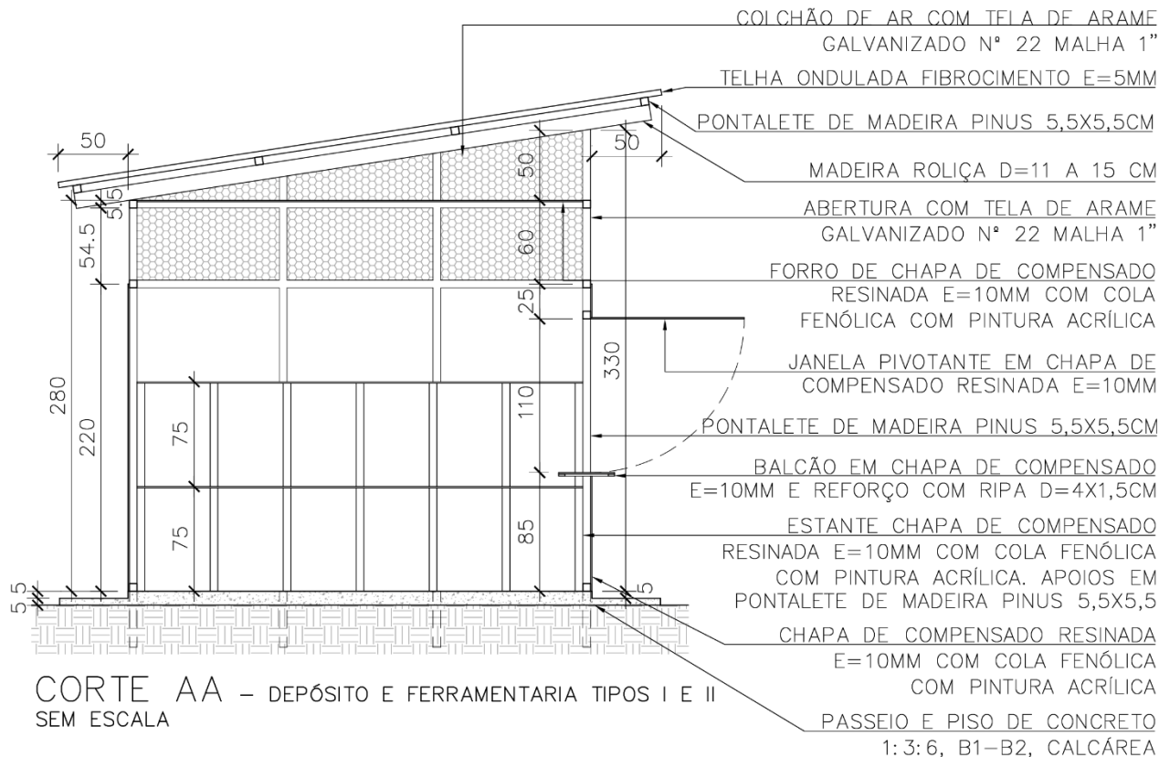
Figura 23 - Corte depósito e ferramentaria. Fonte: Elaboração própria. Nota: Desenho elaborado em 27/09/2024.
