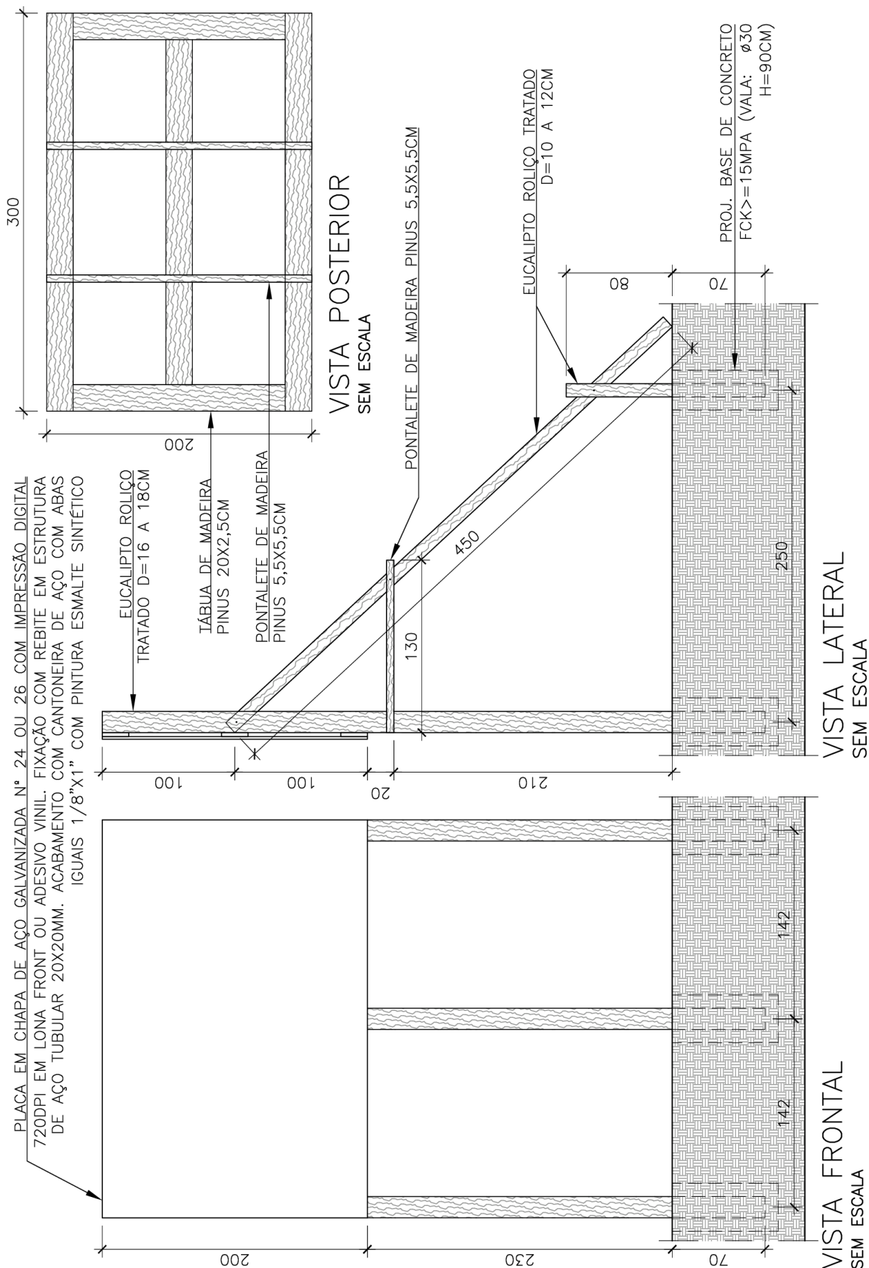
Figura 40 - Placa provisória com informes Sudicap/PBH. Fonte: Elaboração própria. Nota: Desenho elaborado em 30/12/2021.
