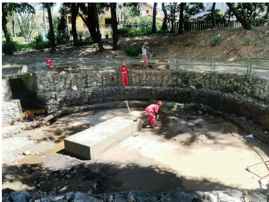
Bacia de Detenção do Córrego Lagoa do Nado (Venda Nova)
