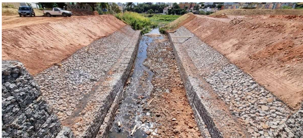
Bacia de Detenção do Córrego Lagoa do Nado (Venda Nova)
