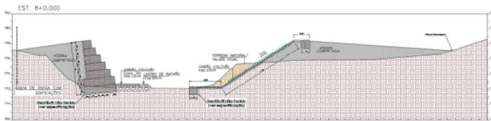
Tratamento da margem esquerda em gabião tipo caixa e na margem direita em gabião tipo colchão com plantio de capim vetiver
