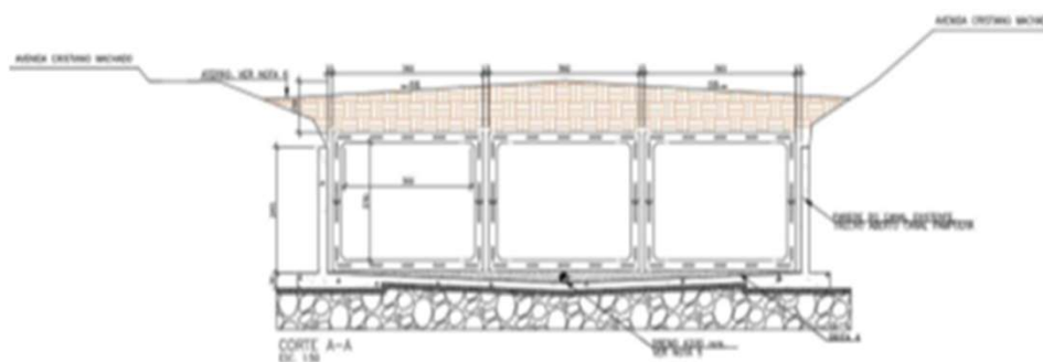
Seção típica do tamponamento provisório do canal existente do Ribeirão Pampulha na Avenida Cristiano Machado durante a execução das obras para permitir os desvios de trânsito.
