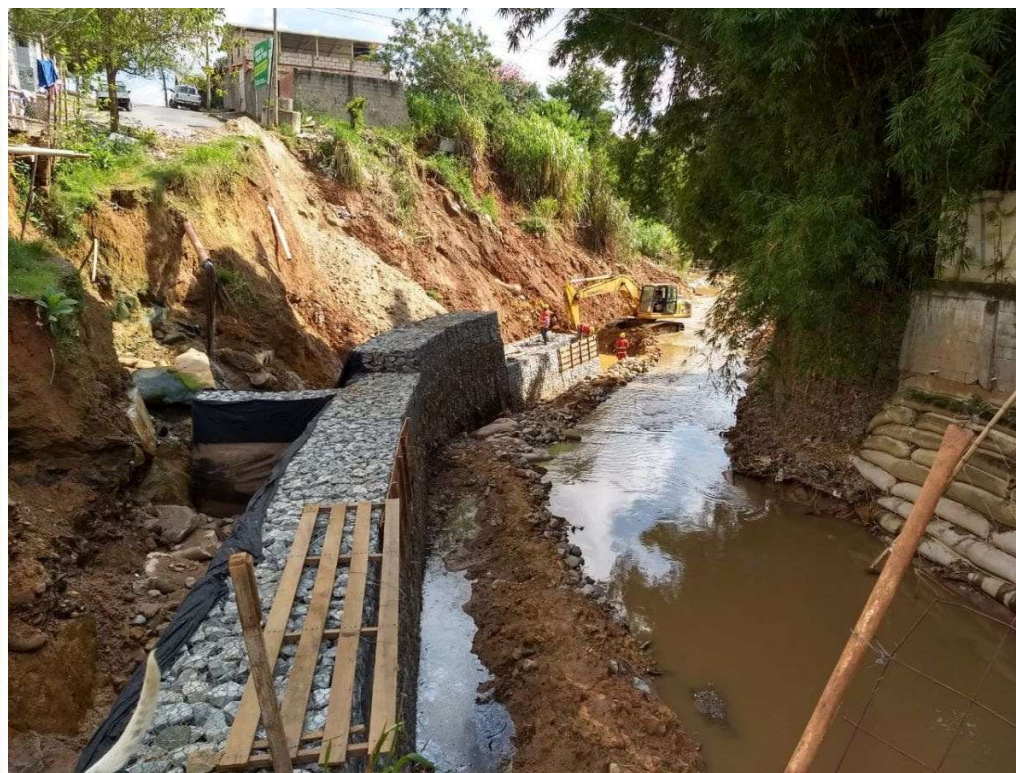
Contenção de margem do Córrego Cercadinho - Rua das Orquídeas com Rua das Espatódias
