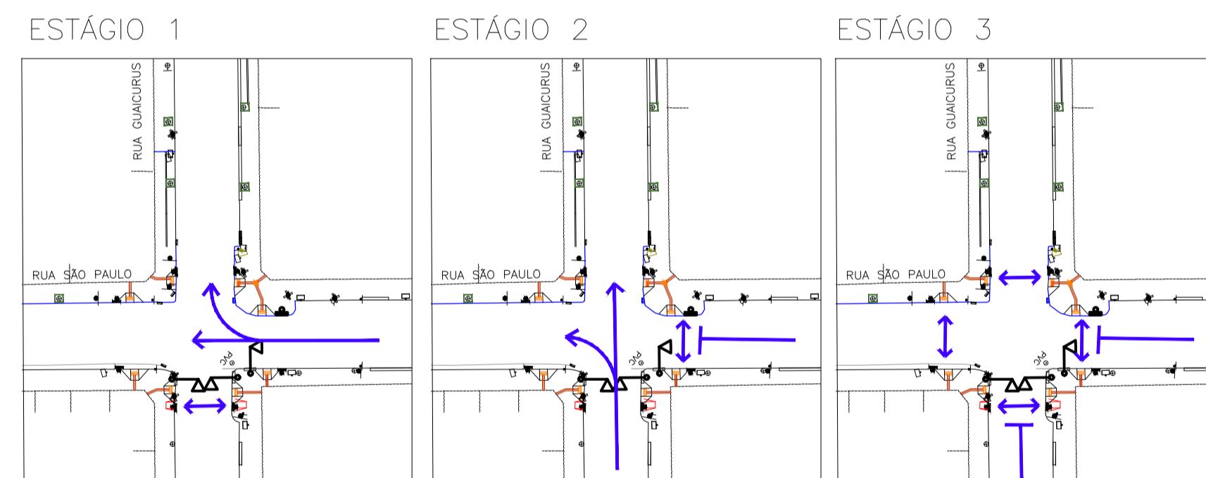
DIAGRAMA DE ESTÁGIOS INTERSEÇÃO: RUA SÃO PAULO x RUA GUACURUS
