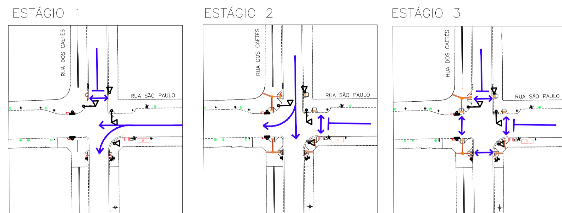
DIAGRAMA DE ESTÁGIOS INTERSEÇÃO: RUA SÃO PAULO x RUA DOS CAETES
