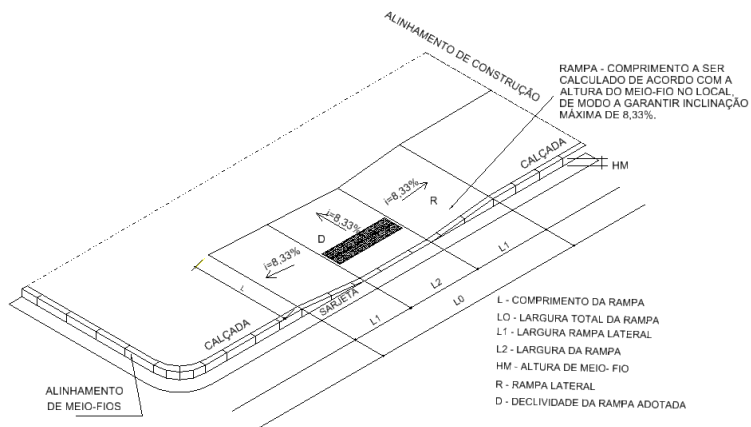
Figura 2 – Perspectiva esquemática rebaixo (Ver padrão ABNT)
