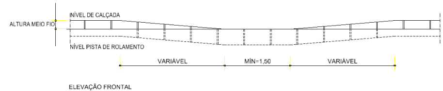
Figura 4 – Elevação esquemática rebaixo (Ver padrão ABNT)
