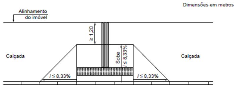
Figura 1 – Planta esquemática rebaixo (Ver padrão ABNT)
