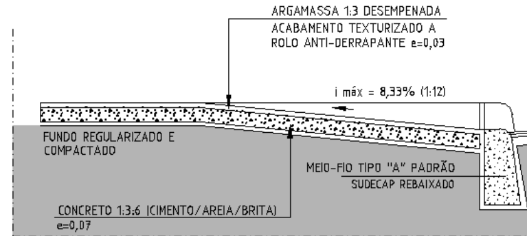
Figura 3 – Corte esquemático rebaixo (Ver padrão ABNT)
