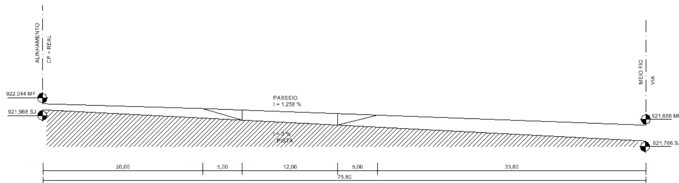
CORTE E-E ESC. 1:25
