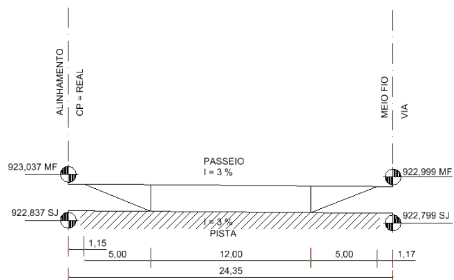
CORTE A-A ESC. 1:25
