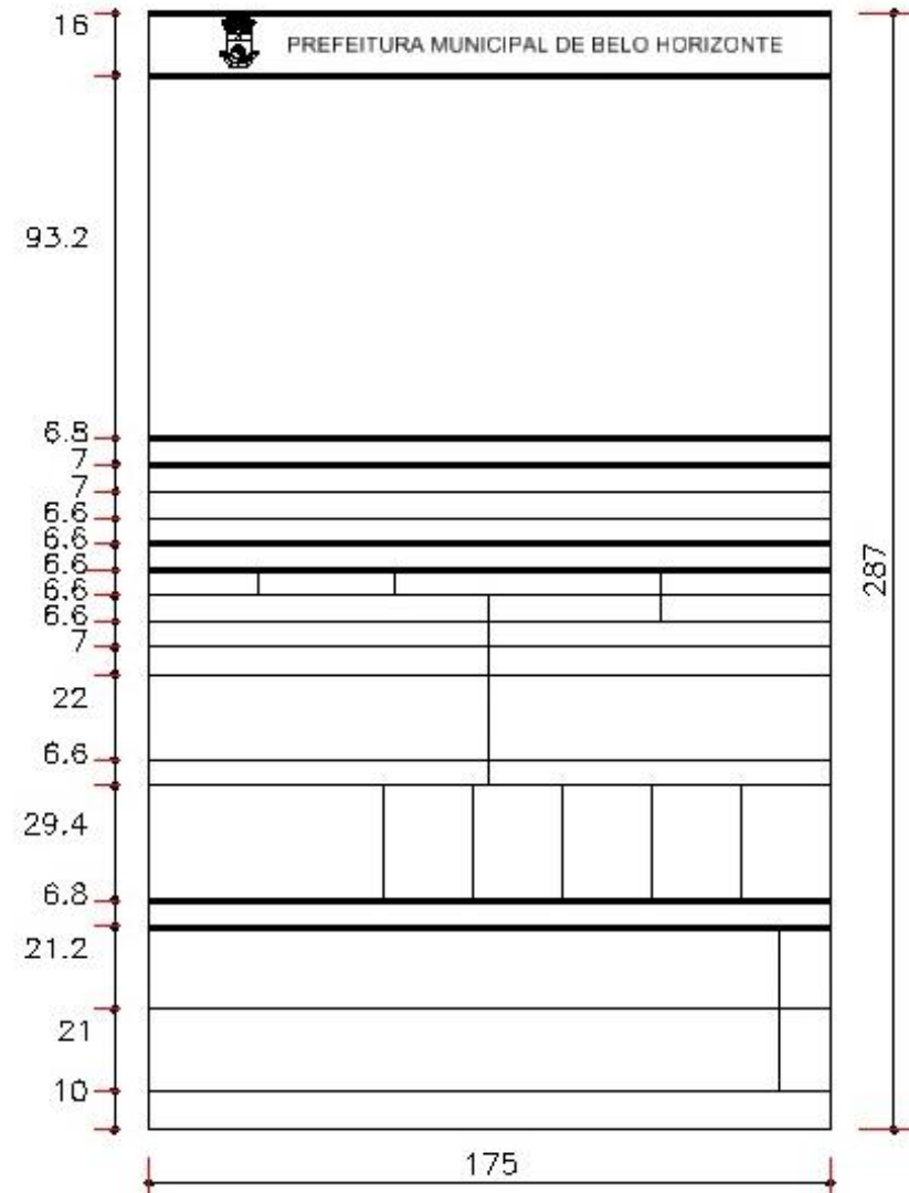
Figura 03 – Cotas básicas do selo padrão PBH
