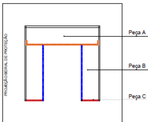
BASE DA ESTRUTURA DA BARRACA ESCALA 1/50
