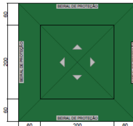
PLANTA DE COBERTURA BARRACA 2,00m X 2,00m
