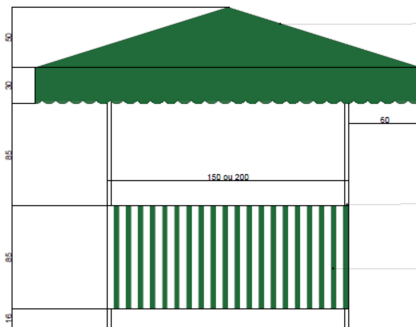
ELEVÇÃO BARRACA ESCALA 1/25
