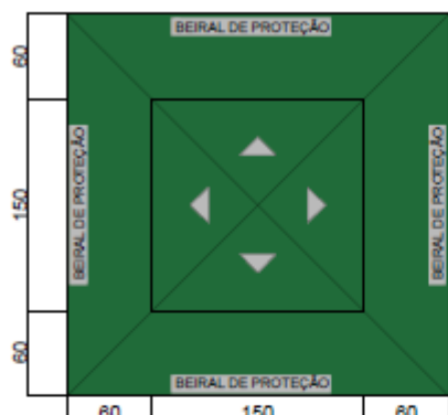
PLANTA DE COBERTURA BARRACA 1,50m X 1,50m
