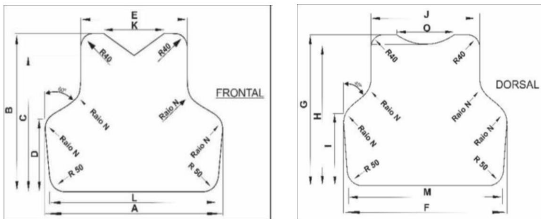
Figura ilustrativa 1: Dimensões do painel balístico
